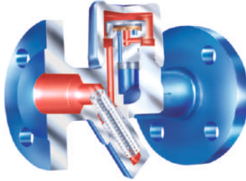
Termostatik ve Termodinamik Kondenstoplar
