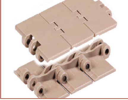
Asetal Palet Bantlar
