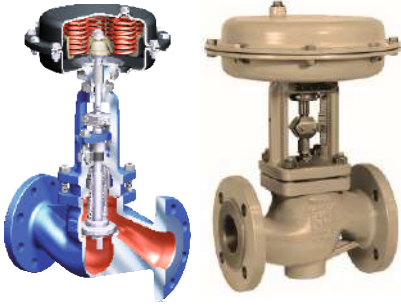
Pnömatik Kontrollü Vanalar
